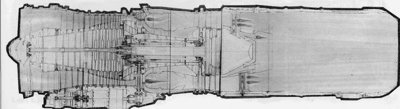
Турбореактивный двигатель АЛ-7Ф
