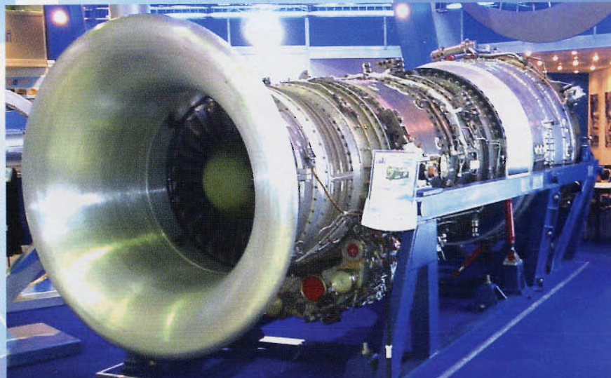
Газотурбинный привод энергоустановки ГТЭ-30-300 на базе двигателя Р79В-300
