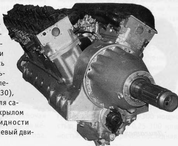
Двигатель АМ-38
